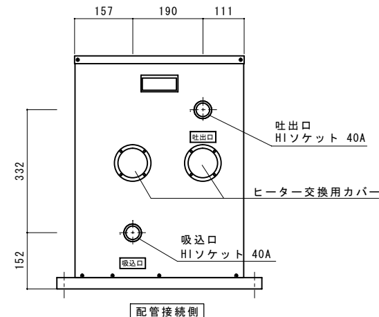
配管接続側
