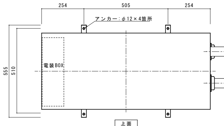
上面
