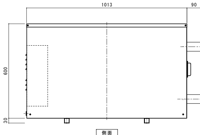
側面
